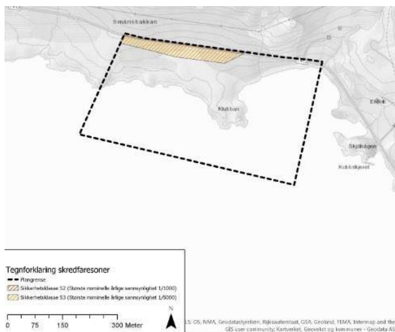
Figur 23. Foreslått skredfaresone
